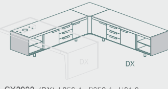
CX2932 (DX) L256,4 P256,4 H61,6 CX2931 (SX) L256,4 P256,4 H61,6
