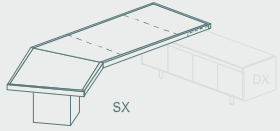
CX2534 (DX) L324,5 P157,4 H75 CX2533 (SX) L324,5 P157,4 H75
