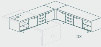
CX2922 (DX) L256,4 P256,4 H61,6 CX2921 (SX) L256,4 P256,4 H61,6
