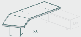
CX2532 (DX) L322,6 P151,7 H75 CX2531 (SX) L322,6 P151,7 H75
